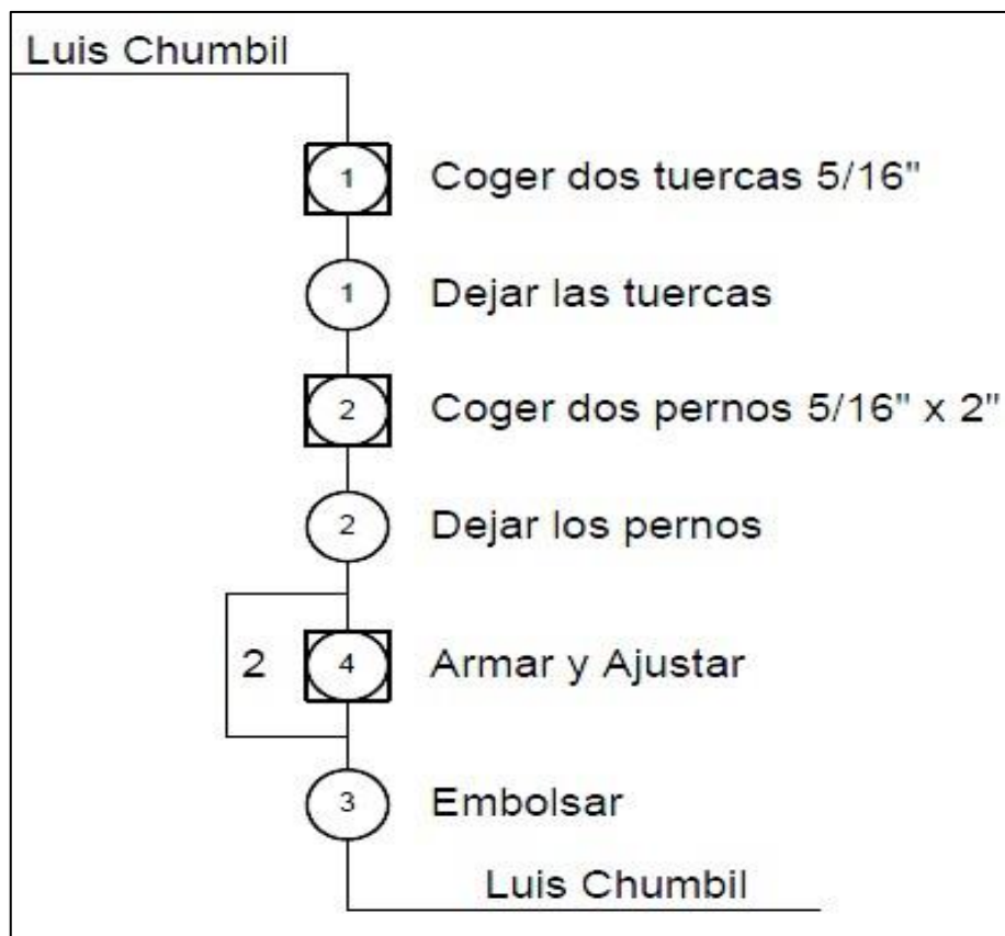
Figura 38. Diagrama de Operaciones (DOP) - Tipo Hombre
