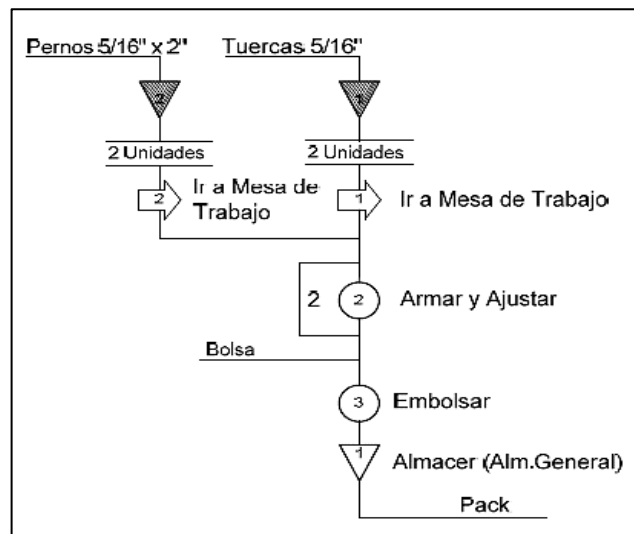
Figura 41. Diagrama de análisis de procesos (DAP) – Tipo Máquina
