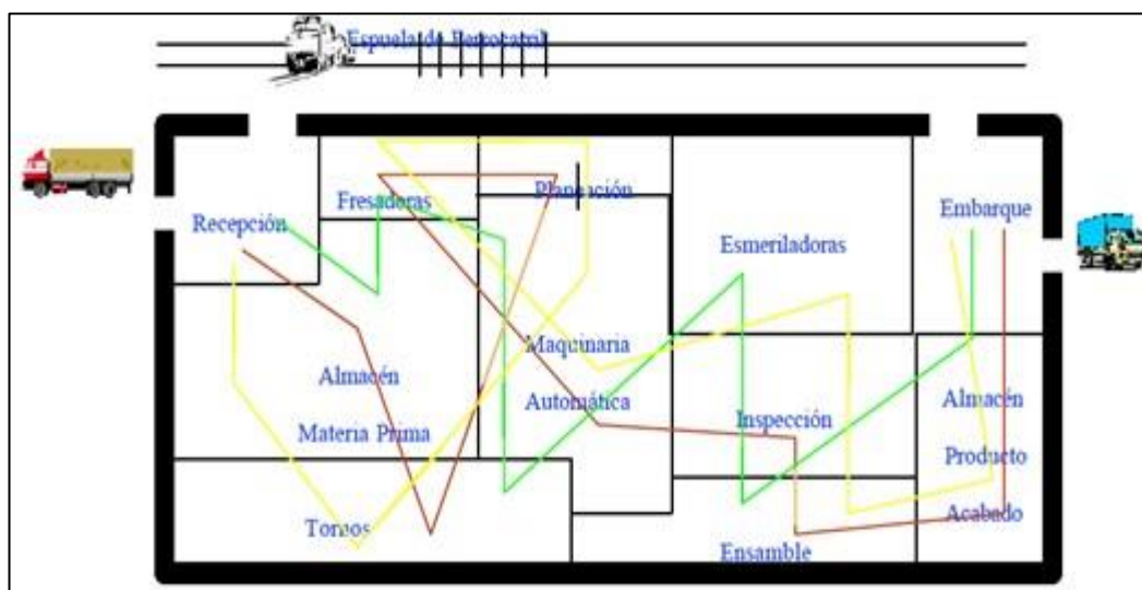
Figura 6. Esquema de Distribución en Planta por Proceso
