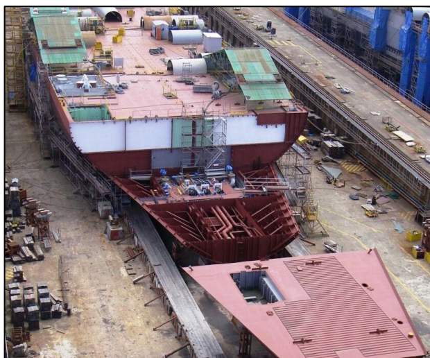
Figura 3. Ensamblaje de Bloques del LHD Juan Carlos I – Ubicación Fija
