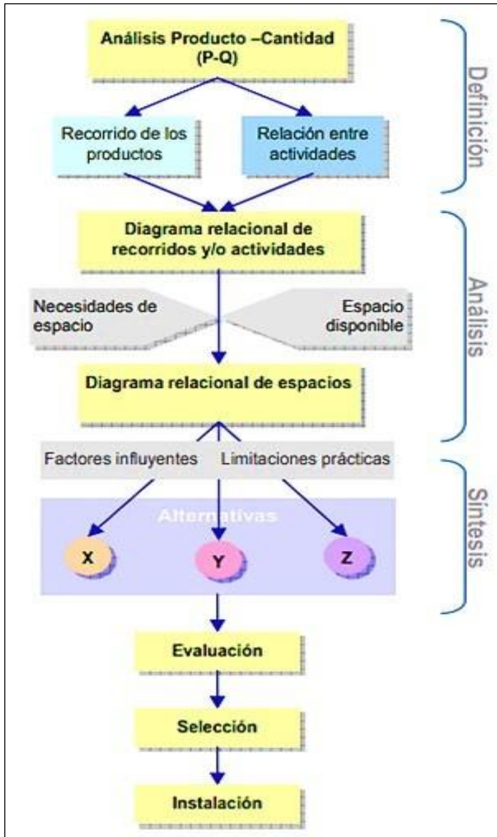
Figura 52. Diagrama análisis P-Q
