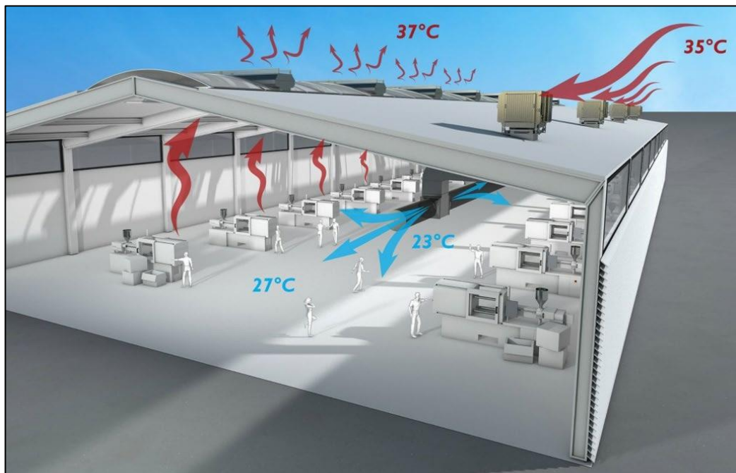
Figura 92. Ventilación por techos
