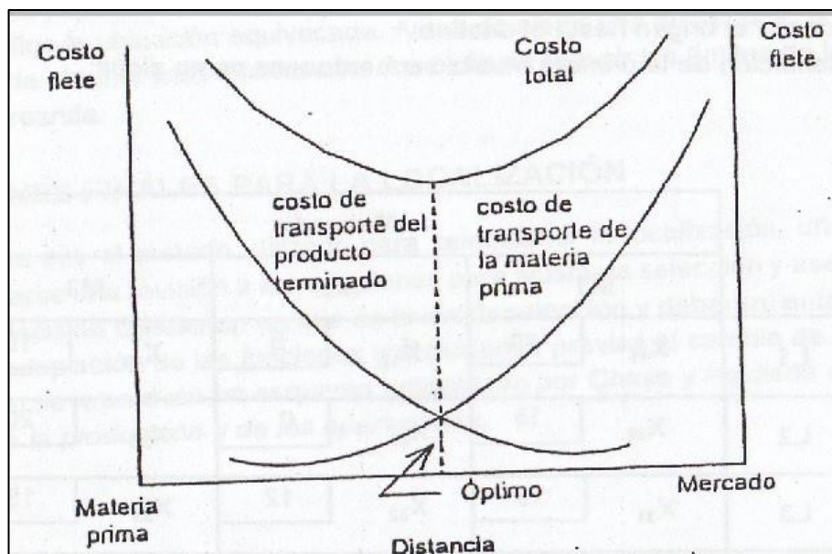
Figura 28. Evaluación e transporte
