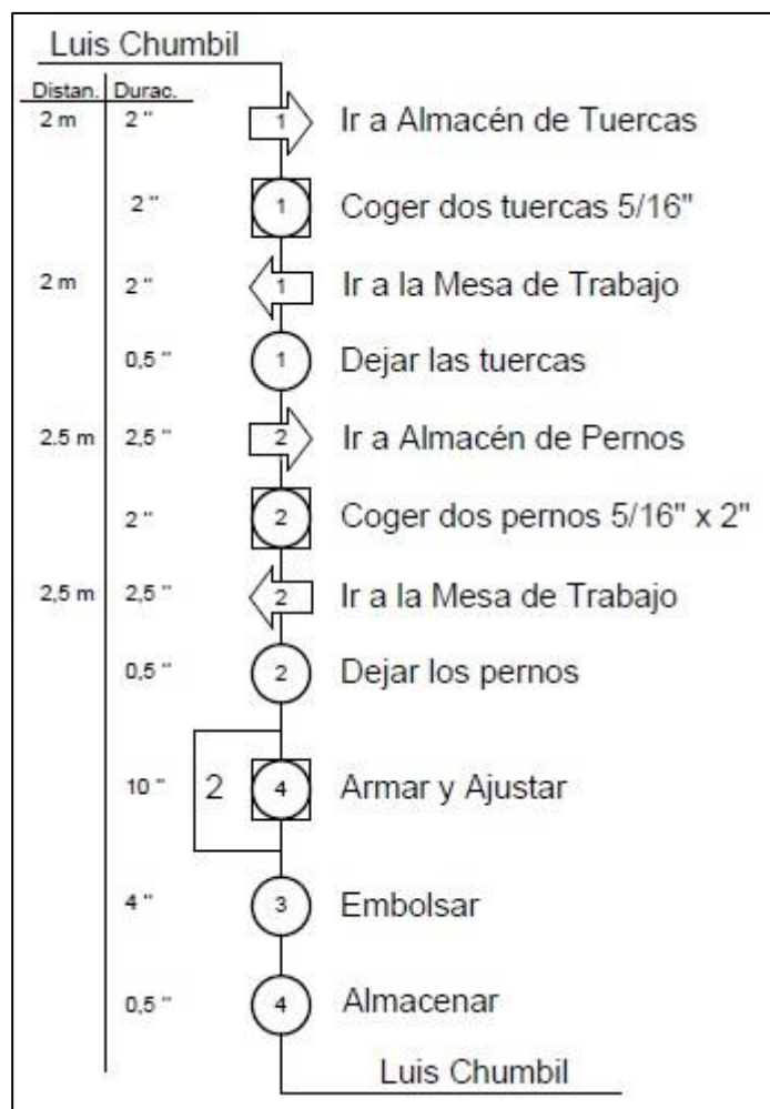
Figura 40. Diagrama de análisis de procesos (DAP) – Tipo Hombre
