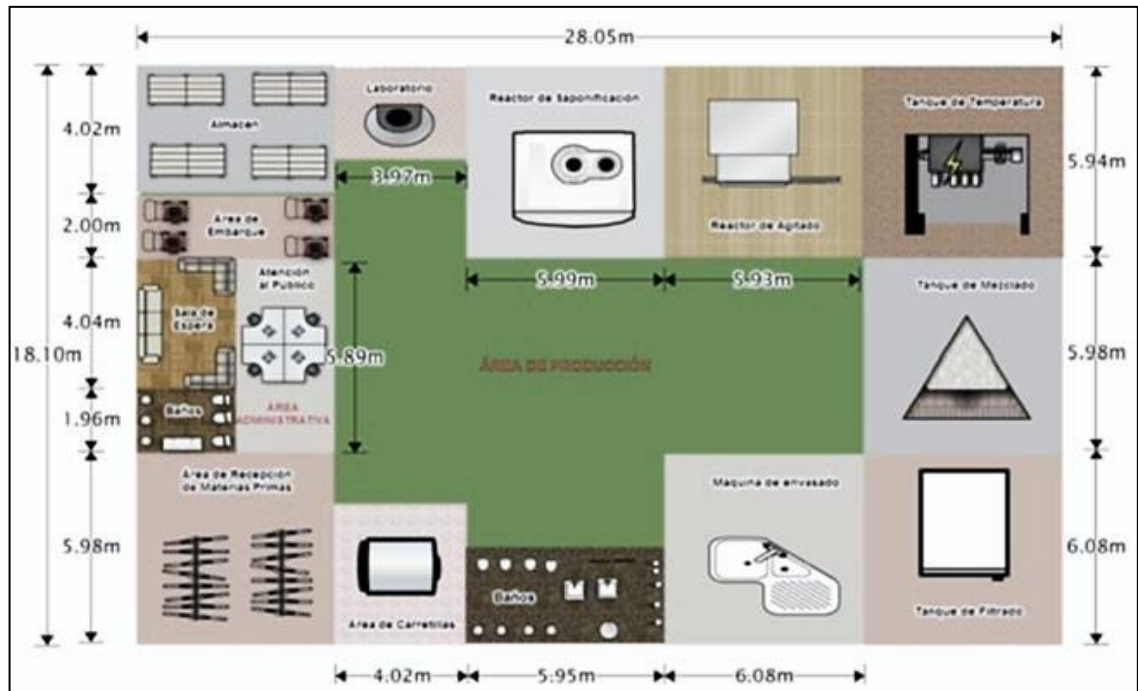
Figura 74. Disposición ideal de una planta productora de jabones
