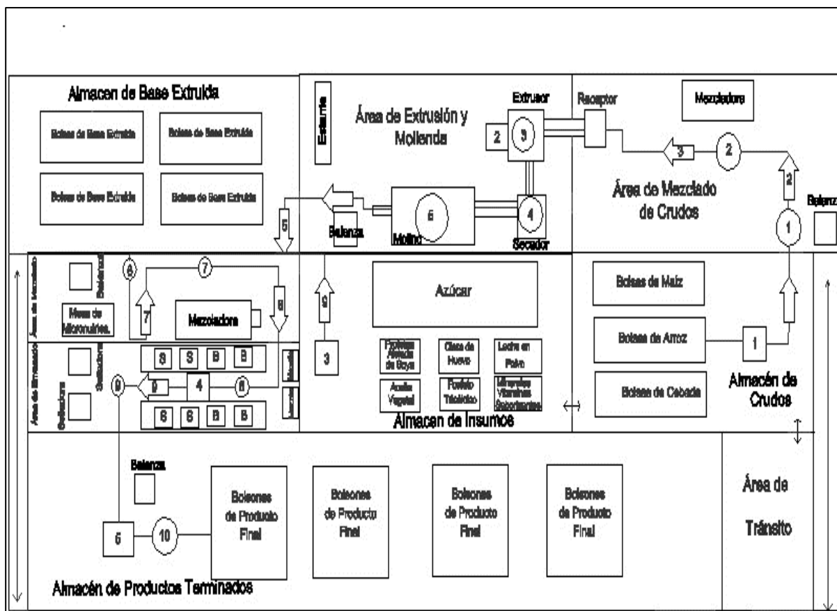
Figura 77. Ejemplo de una distribución a detalle de una planta industrial
