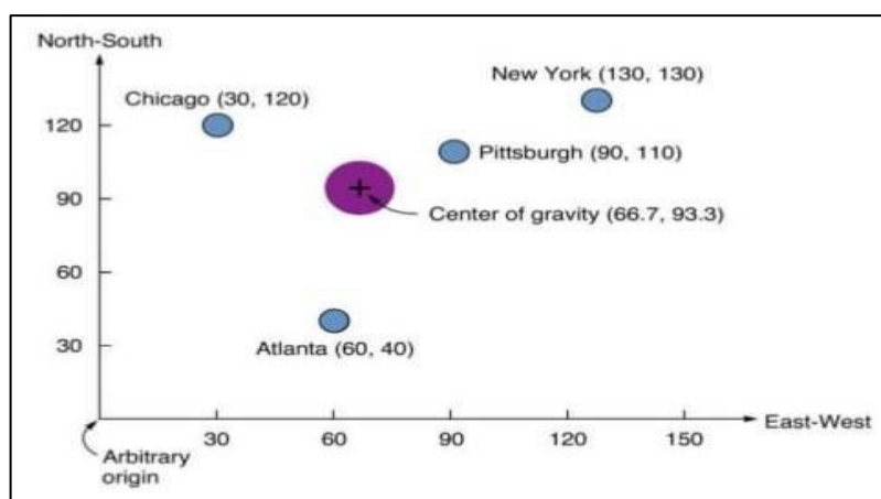
Figura 27. Método del centro de gravedad
