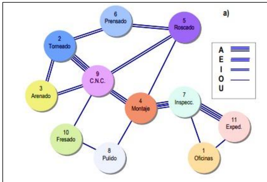
Figura 37. Diagrama Relacional de Espacios
