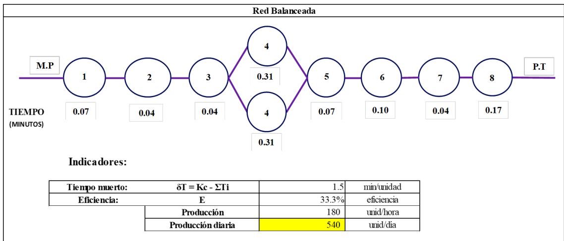
Figura 33. Balance de línea
