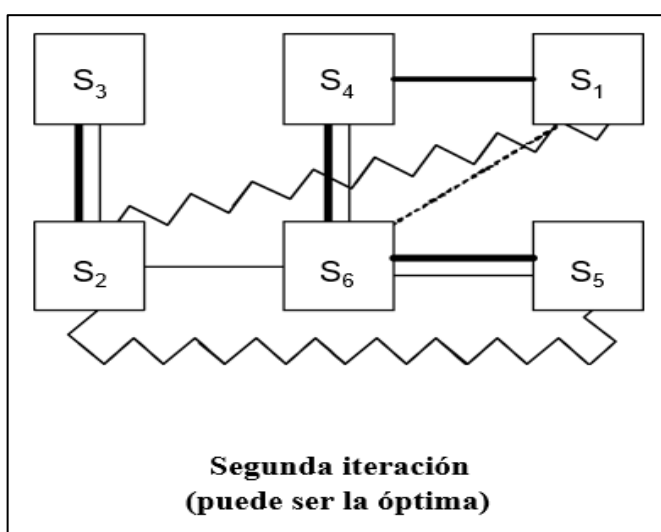
Figura 10. Segunda Iteración de la Gráfica con Cercanías
