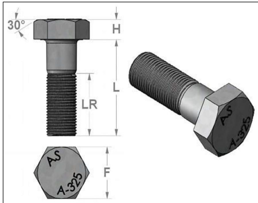
Figura 48. Diseño de un Perno Estructural Cabeza Hexagonal ASTM A-325
