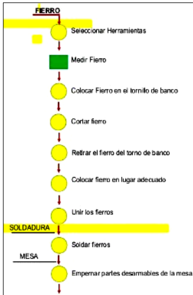
Figura 50. Diagrama de operaciones de la producción
