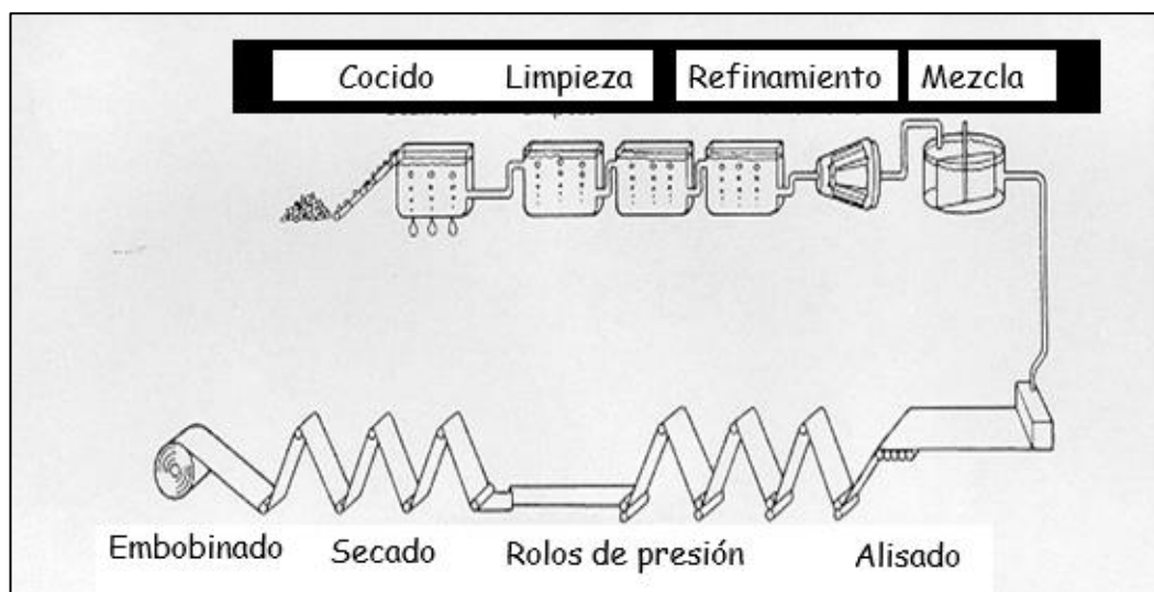
Figura 13. Secuencia del Proceso de Manufactura del Papel
