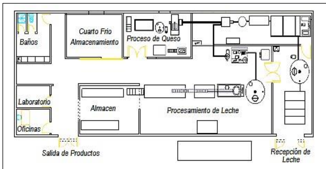
Figura 76. Disposición ideal de una planta productora de quesos
