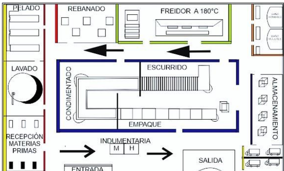
Figura 75. Disposición ideal de una planta productora de papas fritas
