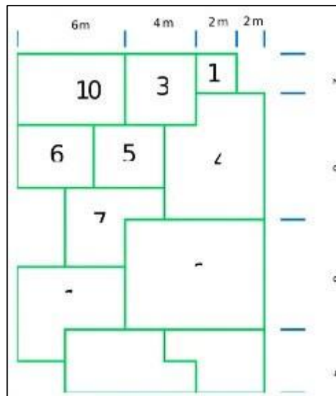
Figura 45. Diagrama de Disposición Ideal
